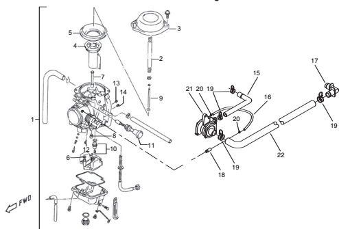
TAV.1 Carburatore - Carburettor - Carburateur - Vergaser - Carbador
