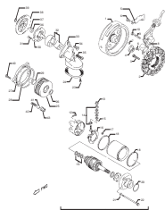
TAV.07-08-10 Pompa olio/Volano magnete/Gruppo accensione elettronica - Oil pump/Flywheel magneto/Electronic ignition assy. - Pompe d'huile/Volant magnetique/Groupe allumage electronique - Olpumpe/Lichtmaschine/Elektronischezündung gruppe - Bomba de aceite/Volante magnetico/Grupo encendido electrónico
