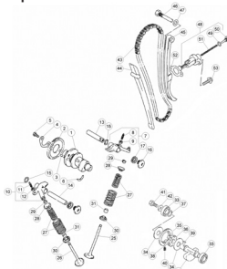
TAV.11B Albero a camme-valvole - Camshaft-Valves - Arbre à cames-Soupapes - Nockenwelle-Ventil - Eje de excentricas-Válvulas
