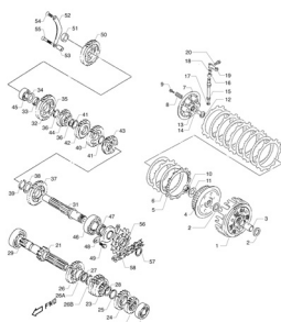
TAV.03-04 Frizione/Ingranaggi cambio - Clutch/Gear group - Embrayage/Engrenages changement de vitesses - Kupplung/Schaltgetriebe - Embrague/Engranaje del cambio
