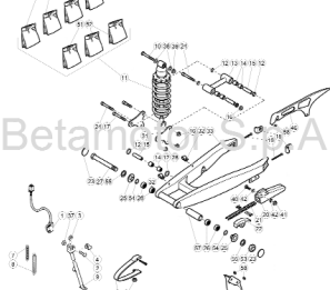
TAV.33 Sospensione posteriore/Forcellone - Rear suspension/Rear fork - Suspension arrière/Fouche arrière - Hinterfederung/Hinterradschwinge - Suspensión trasera/Horquilla posterior
