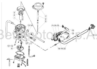
TAV.12 Carburatore - Carburettor - Carburateur - Vergaser - Carburador
