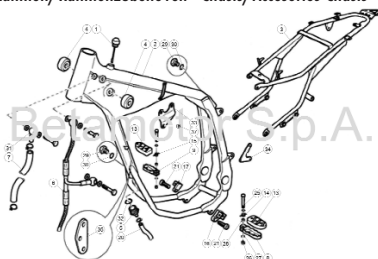
TAV.31-32 Telaio/Accessori telaio - Frame/Frane accessories - Chassis/Accessoires chassis - Rahmen/Rahmenzubehör en - Chasis/Accesorios Chasis
