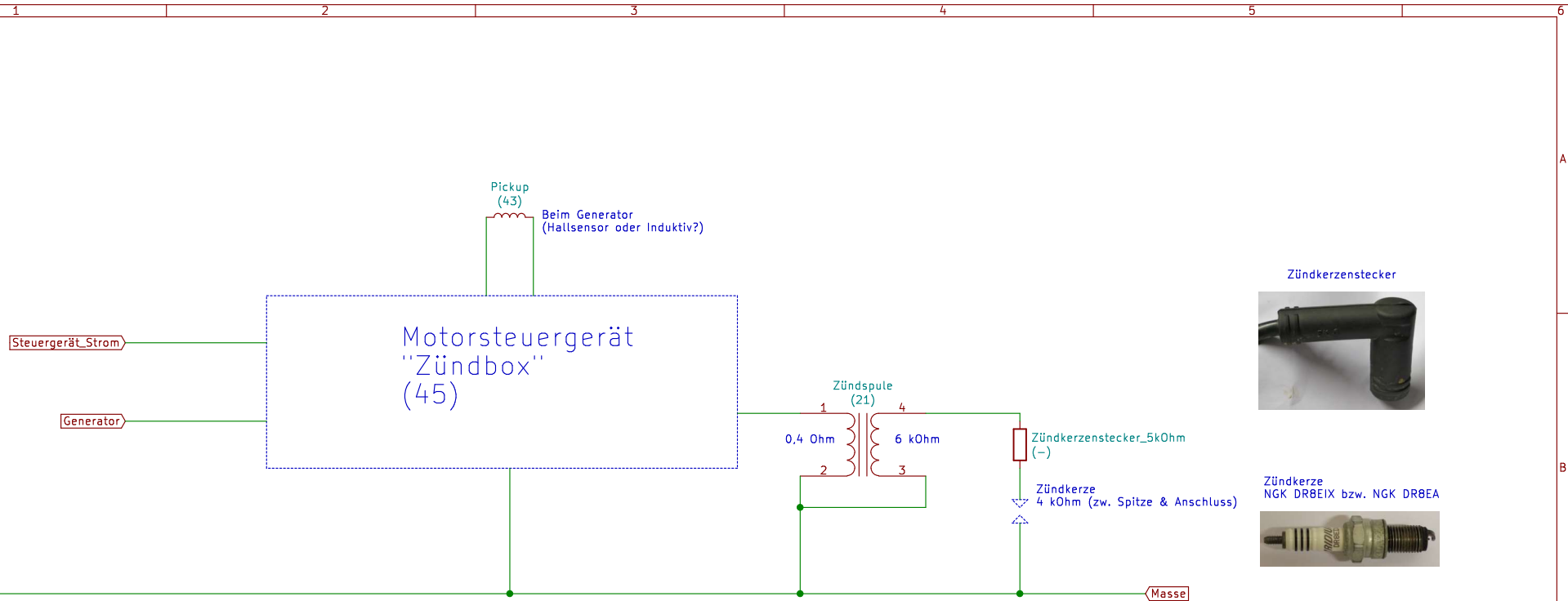
Motorsteuergerät
