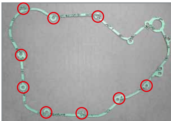
Positionierung der Schrauben M6x25.
