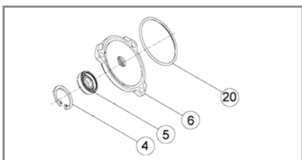
Explosionszeichnung der Öldruckpumpe. 4) Seegering JS24; 5) Wellendichtring 10x22.6; 6) Deckel der Ölpumpe; 20) O-Ring 45x2
