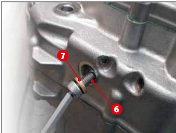
Schraube 6, die die Kurbelwelle blockiert, mit Unterlegscheibe aus Kupfer 7.
