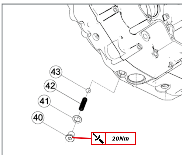
Verbindung des Deckels der Druckpumpe mit dem Gehäuse.
