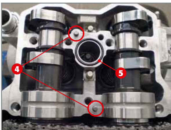
Die beiden Zentrierstifte 4 und der O-Ring 5 um den Kerzenschacht.
