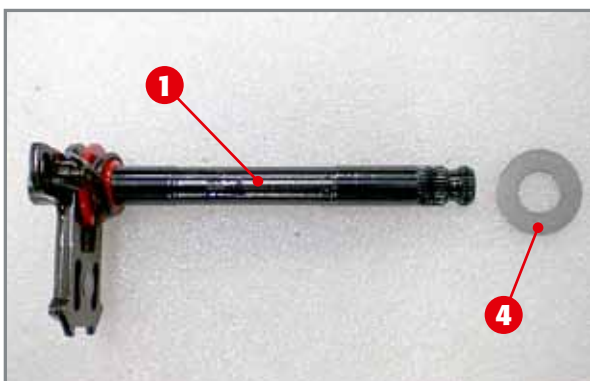
Die Schaltwelle mit Unterlegscheibe.
