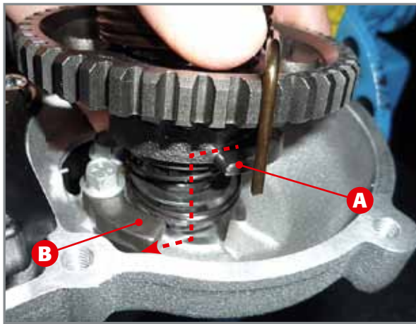
Positionierung des Sperrrades A unter der Rampe B.
