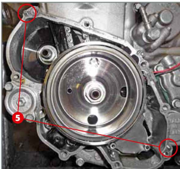
Die beiden Zentrierstifte 5 für den Schwungraddeckel.
