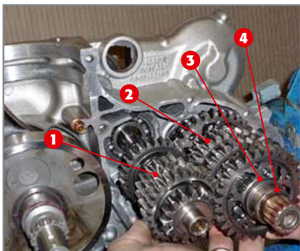
Einsetzen des Getriebes in die linke Gehäusehälfte.
