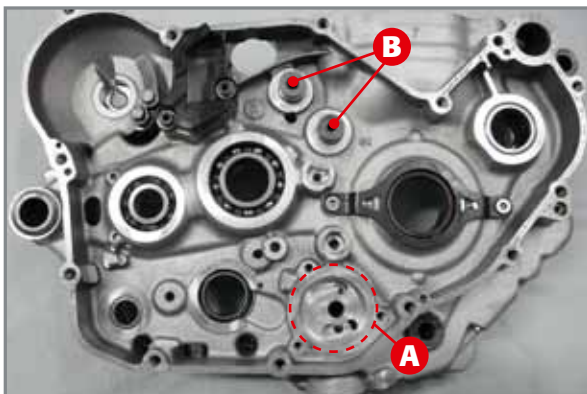
Vorrichtung zur Gangarretierung, die mit der Gehäusahälfte verbunden ist.
