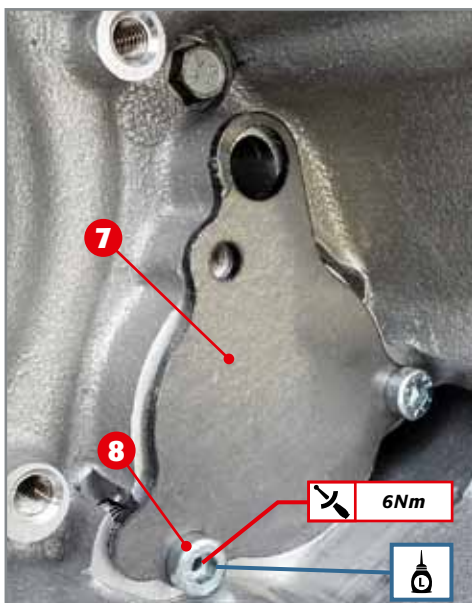
Verbindung des Deckels der Absaugpumpe mit dem Gehäuse.
