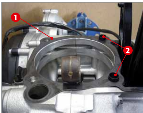
Anbringen der Dichtung zwischen Zylinder und Gehäuse und der Passbüchsen.
