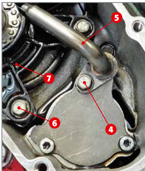
Kettenschutz und Spritzdüse.
