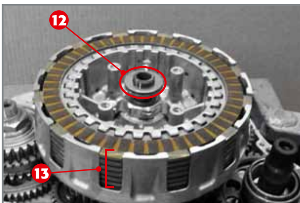
Druckpilz 12 und Kupplungsscheibenpaket 13.
