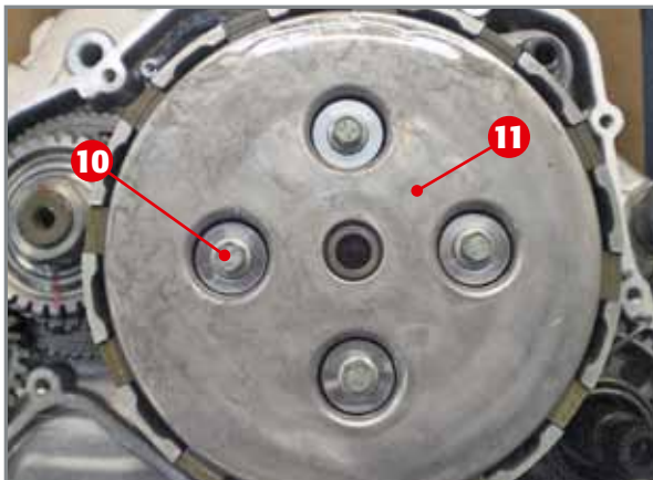
Die Druckkappe 11 und die vier Schrauben 10.
