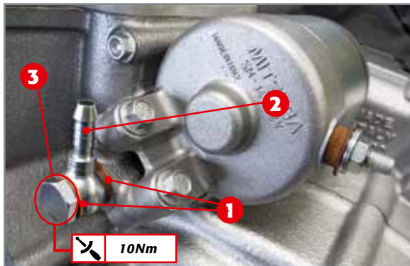
Die Entlüftungsvorrichtung für die Öldämpfe des Getriebes.
