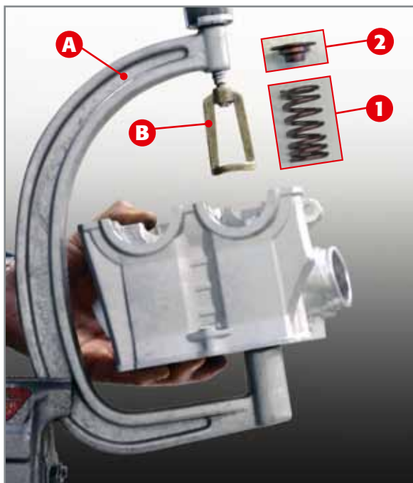
Platzierung des Kopfes auf dem Ventil-Montagewerkzeug.
