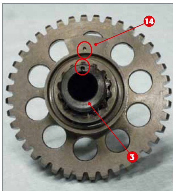
Positionierung des Sperrrades auf der Welle.
