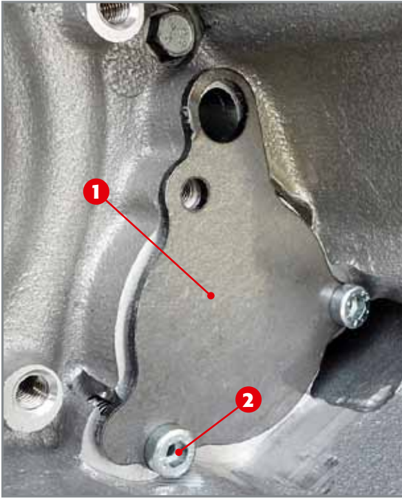
Deckel und Schrauben der Saugpumpe.
