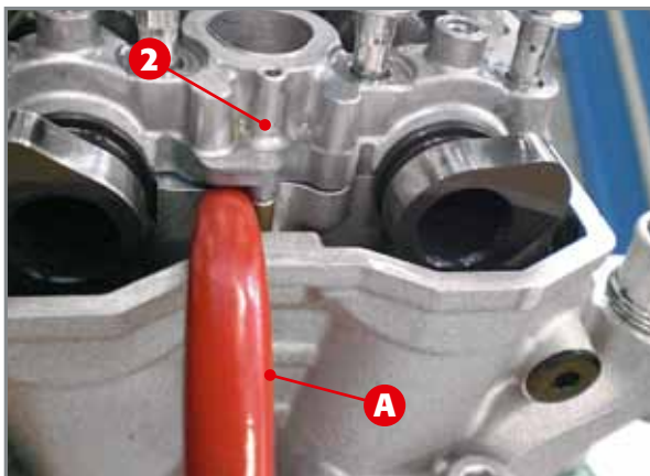
Anheben der Lagerbrücke 4 des Zylinderkopfes.
