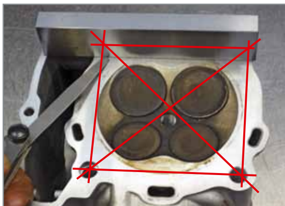
Überprüfung der Ebenheit des Zylinderkopfes.
