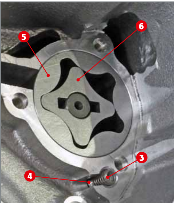
Saugpumpe und By-pass-Ventil.
