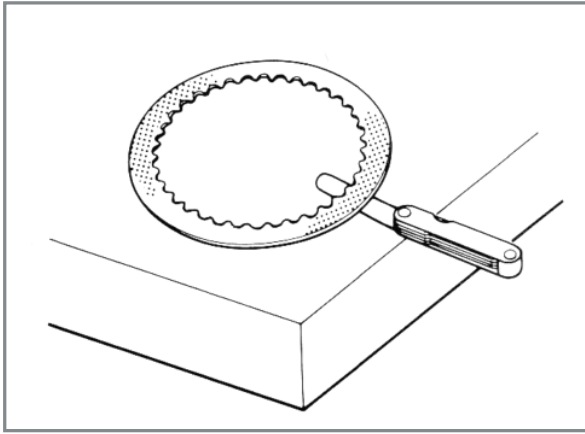
Messung des Verzugs der Stahllamellen.
