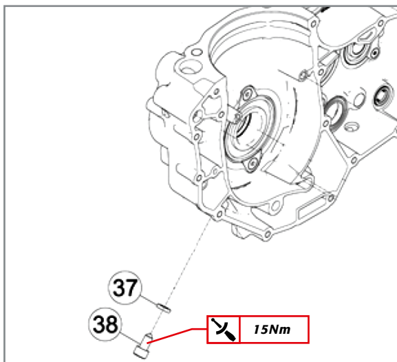
Die Entlüftungsvorrichtung für die Öldämpfe des Getriebes.
