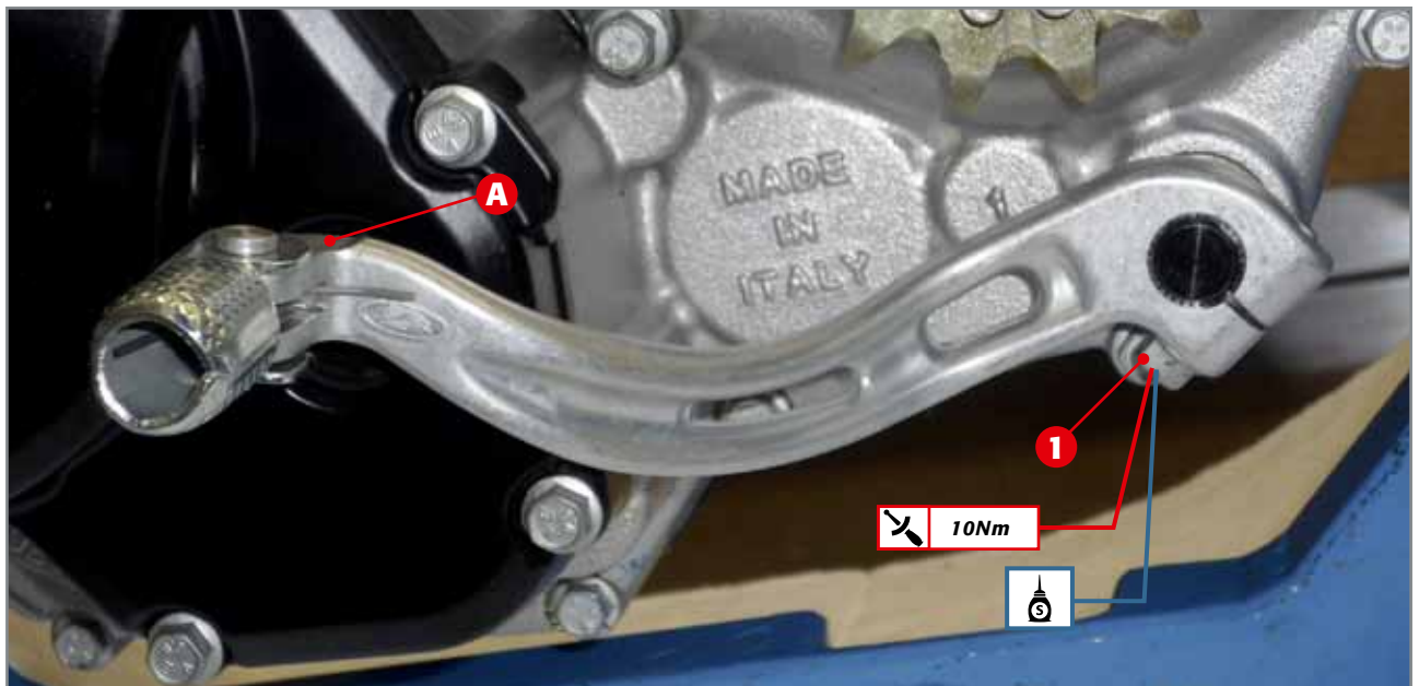
Positionierung des Schalthebels
