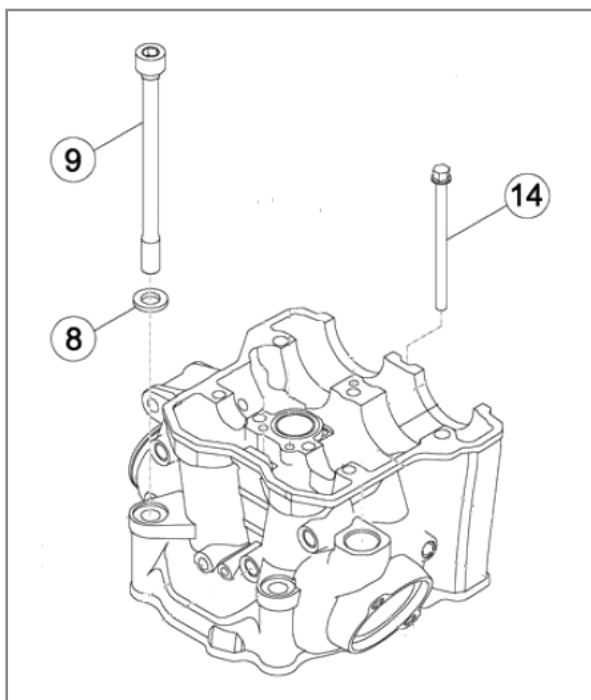
Anbringen der Komponenten für das Verbinden des Kopfes und des Zylinders am Gehäuse.
