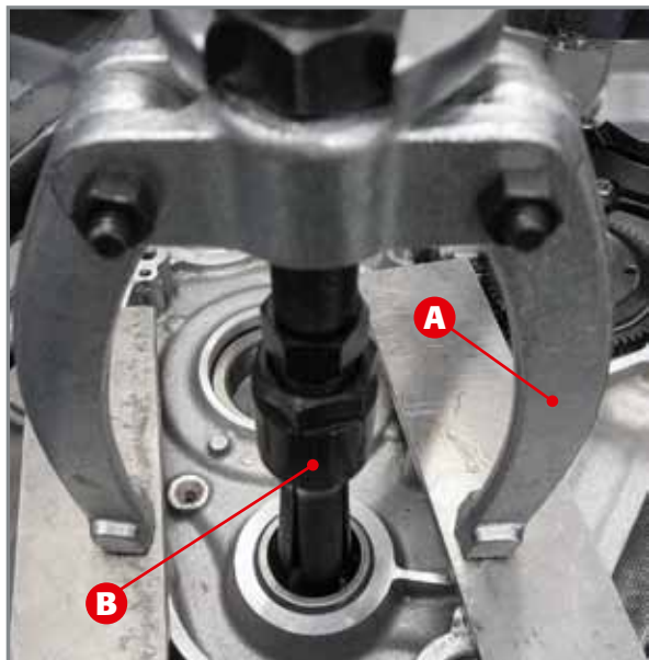
Entfernung des Lagers der Ausgleichswelle.
