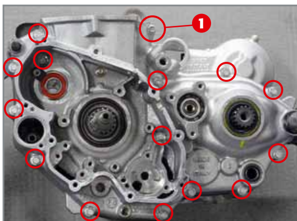
Gehäuseschrauben 1.
