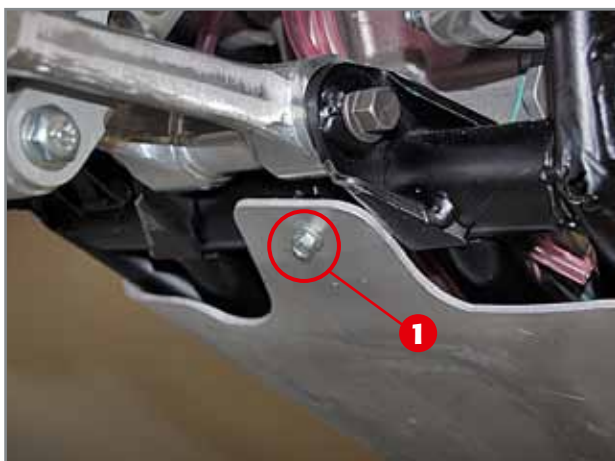
Hintere Befestigungsschraube der Motorschutzabdeckung
