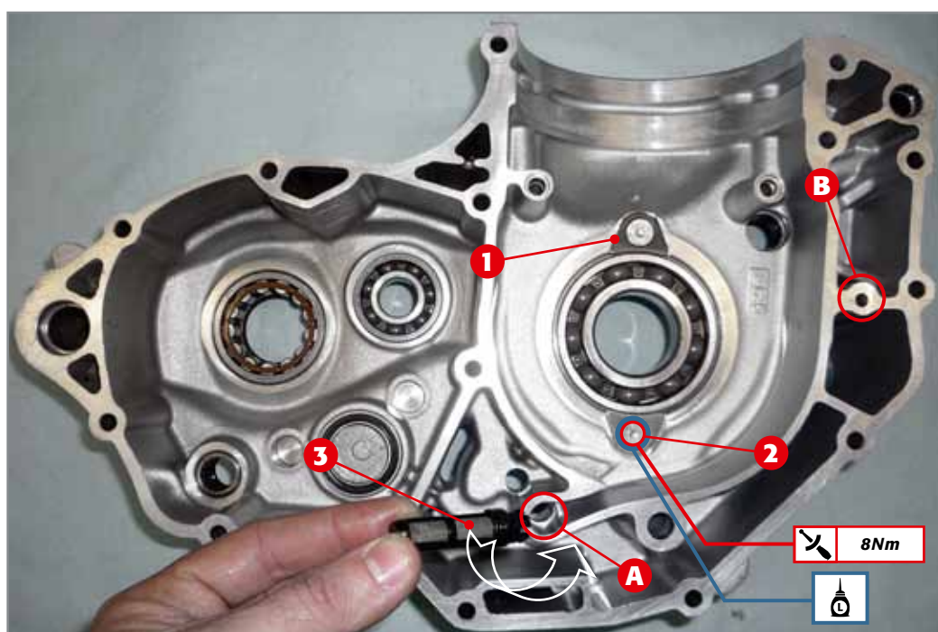
Element an der Innenseite der linken Gehäusehälfte.
