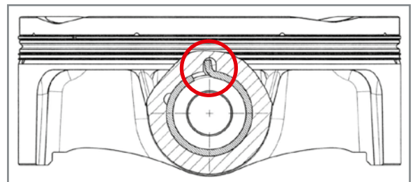
Sitz für Seegernase 350cc.
