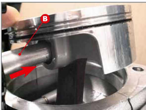
Entfernung des Kolbenbolzens.
