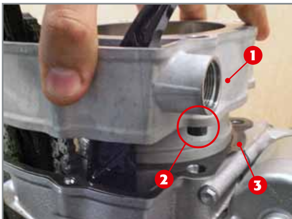
Entfernung des Zylinders.
