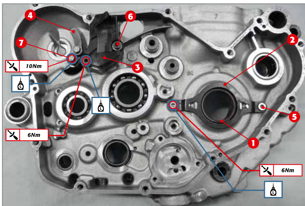
Elemente an der Außenseite der rechten Gehäusehälfte.
