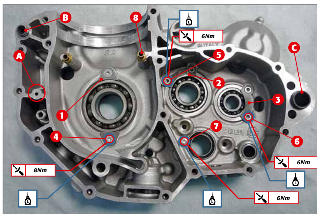
Elemente an der Innenseite der rechten Gehäusenhälfte.
