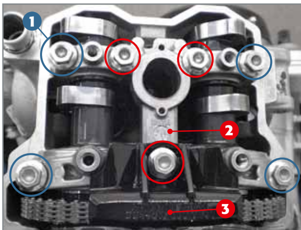
Befestigungsschrauben 1 der Lagerbrücke 2 und die Kettenführung 3. Die vier äußeren Schrauben, die blau umrandet sind, müssen zuerst entfernt werden.
