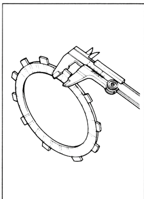
Mindeststärke der Verzahnung der Belaglamellen.
