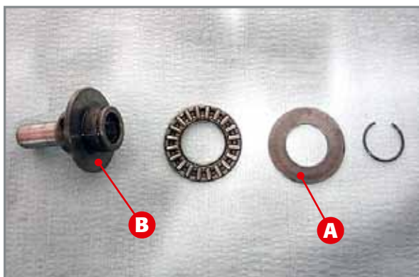
Druckpilz.
