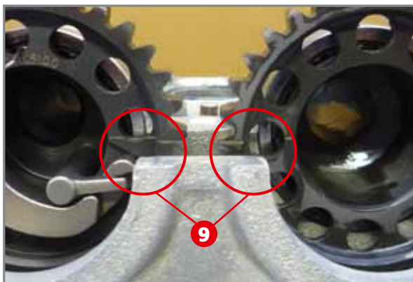
Ausrichtung der Markierungen der Nockenwellen.
