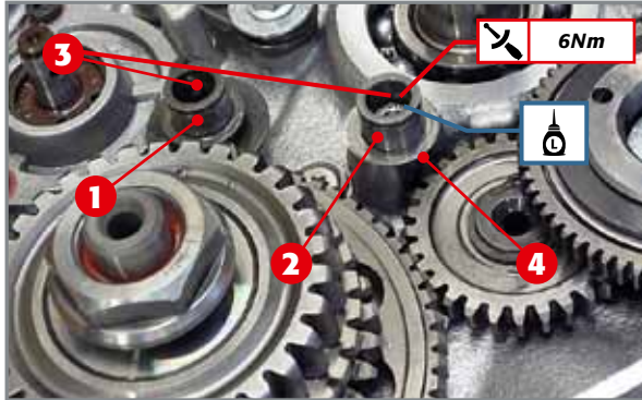
Haltezapfen der Antriebszahnräder der Ölpumpen.
