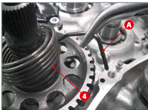
Aushängen der Feder aus dem Gehäuse.
