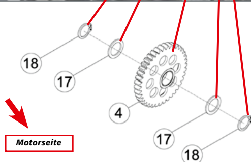
Kickstartervorrichtung im Gehäuse.
