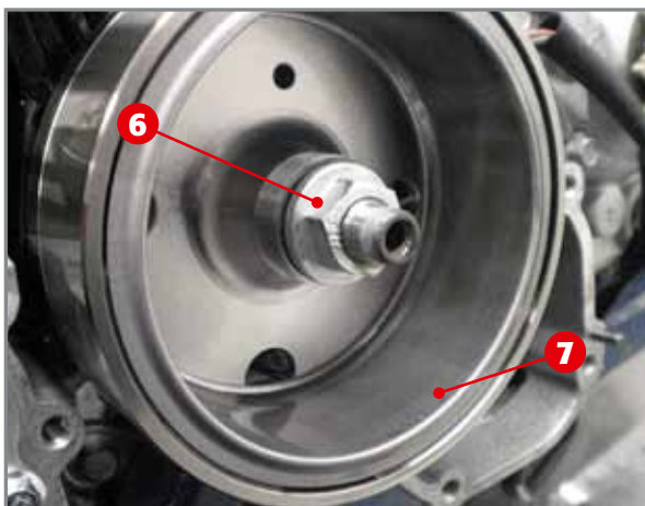
Mutter 6, die das Schwungrad 7 an der Kurbelwelle fixiert.
