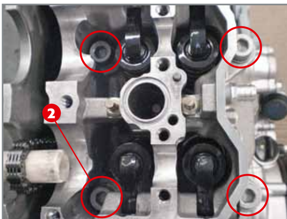
Klemmschrauben des Zylinderkopfes.
