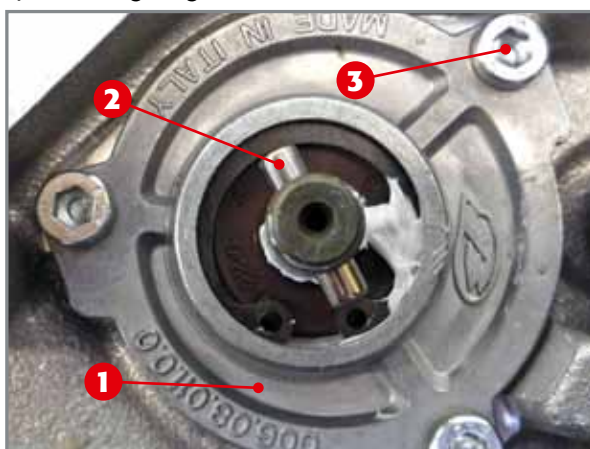
Entfernung des Deckels der Öldruckpumpe.
