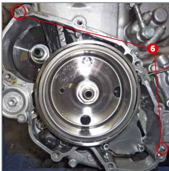
Anbringen der Zentrierstifte an der linken Gehäusehälfte.
