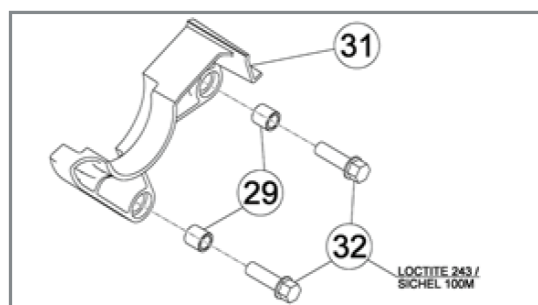
Montage der Buchsen in den unteren Ösen des Kettenschutzes.
