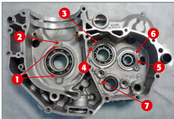
Lagersicherungen an der Innerseite der rechten Gehäusehälfte.
