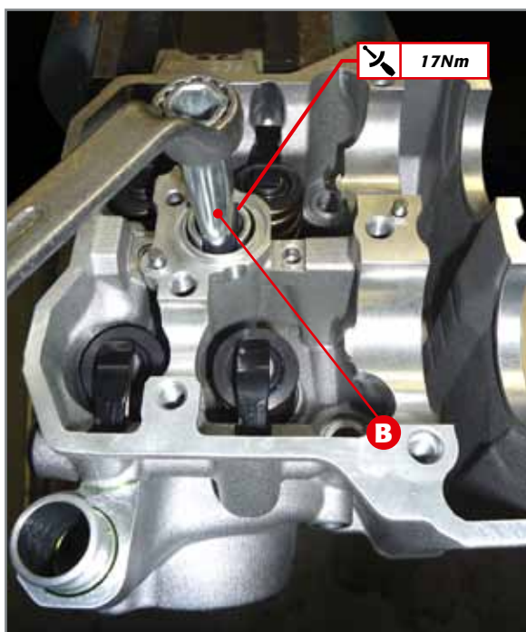
Anbringen der Verschlusschrauben.
