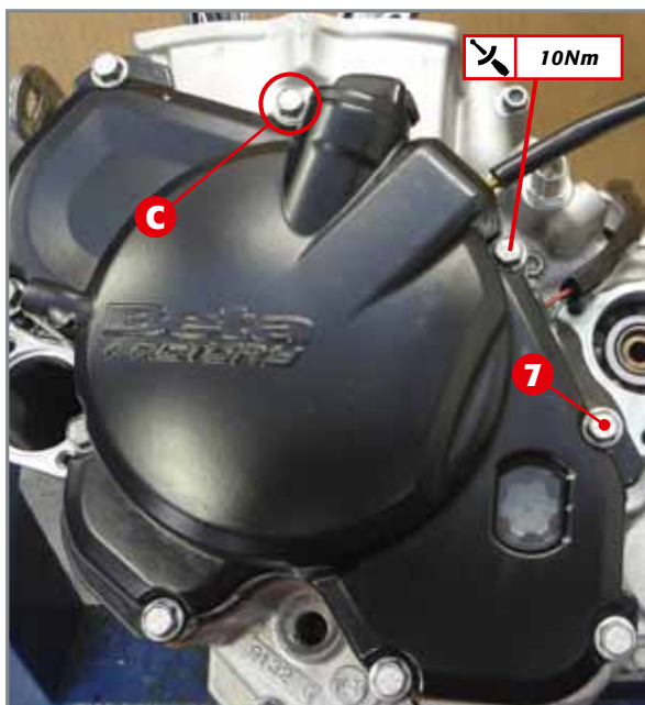
Zündungsdeckel am Gehäuse.
