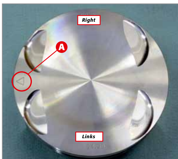
Bestimmung Einbaurichtung.
