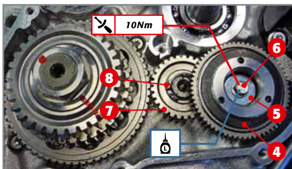
Verbindung des Antriebsstrangs des elektrischen Anlassers.
