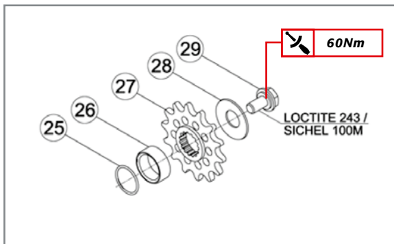
Explosionszeichnung des Ritzels. 25) O-Ring 25x12x1,78; 26) Distanzring; 27) Ritzel; 28) Scheibe; 29) Schraube.
