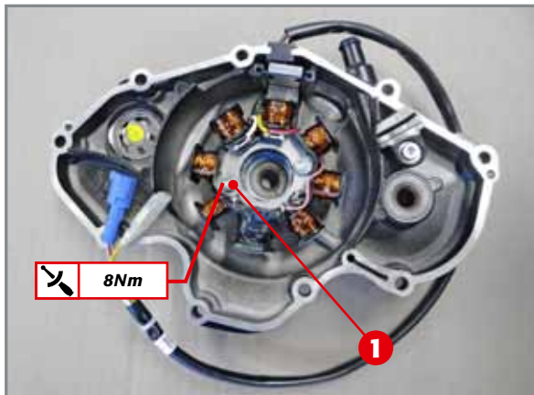
Anbringen des Stators am Zündungsdeckel.
