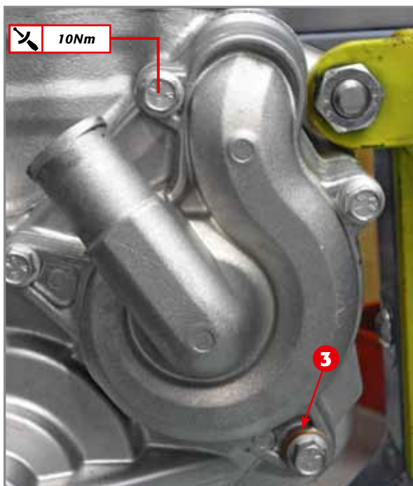
Wasserpumpendeckel: Auf die Kupferscheibe 3 achten.
