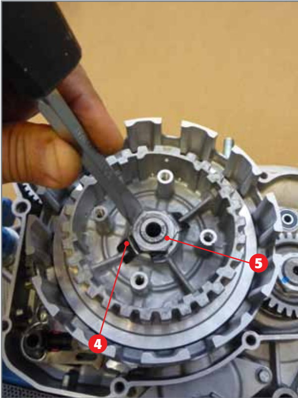
Öffnung der Sicherungsscheibe mit dem Schlitzmeißel
