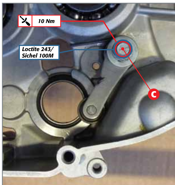
Anbringung Nockenanslagshebel.
