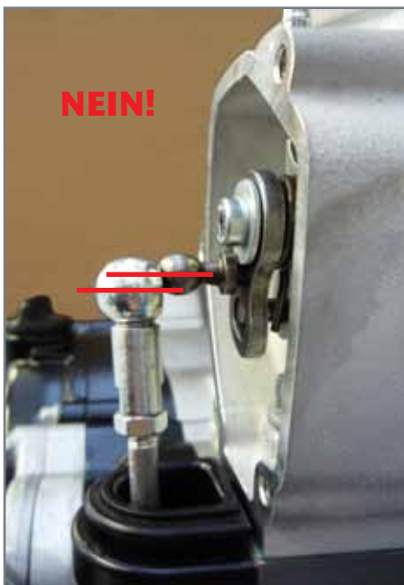
Falsche Stellung des Sitzes der Steuerstange.
