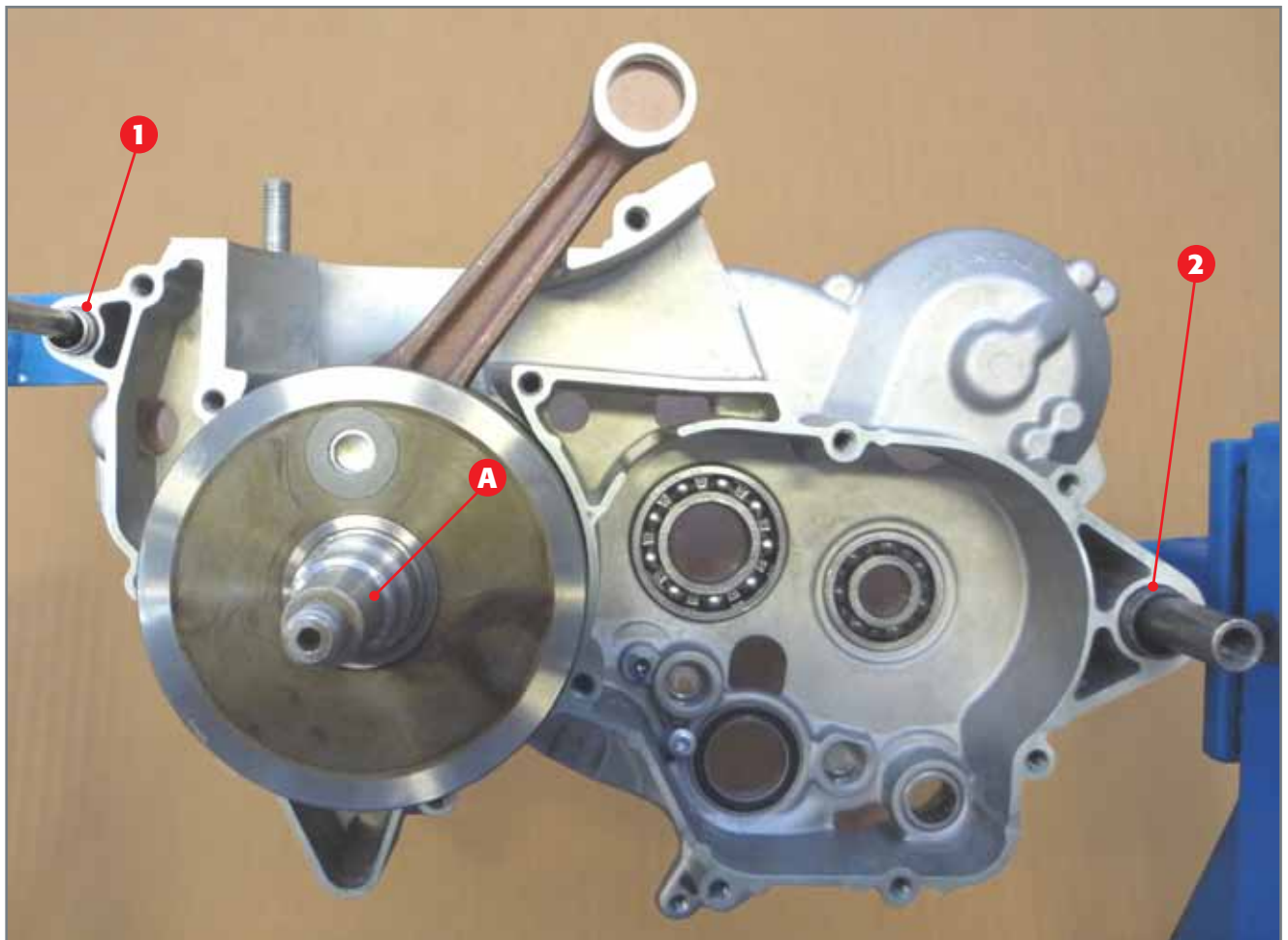
Einsetzen der Kurbelwelle in die rechte Gehäusehälfte.
