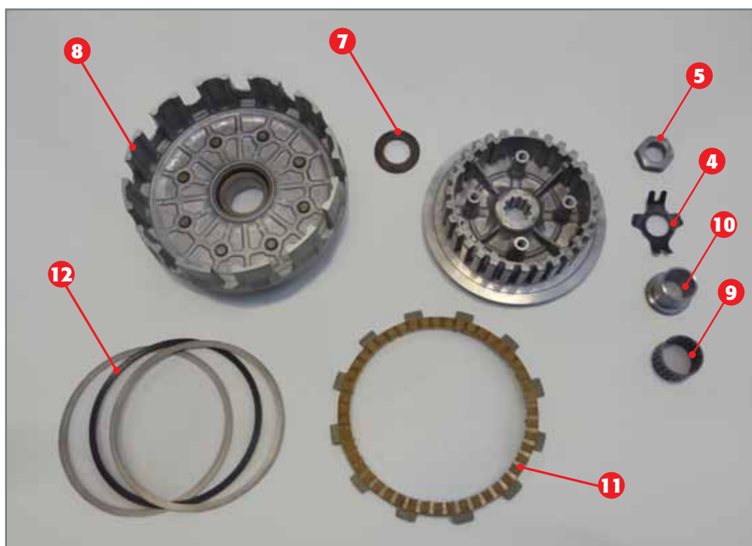
Sicherungsscheibe 4 ; Mutter 5 ; Scheibe 7 ; Kupplungskorb 8 ; Nadelkäfig 9 ; und Lagerschale 10 ; Spezielle Stahlscheibe 11 ; Spannscheibe 12 .
