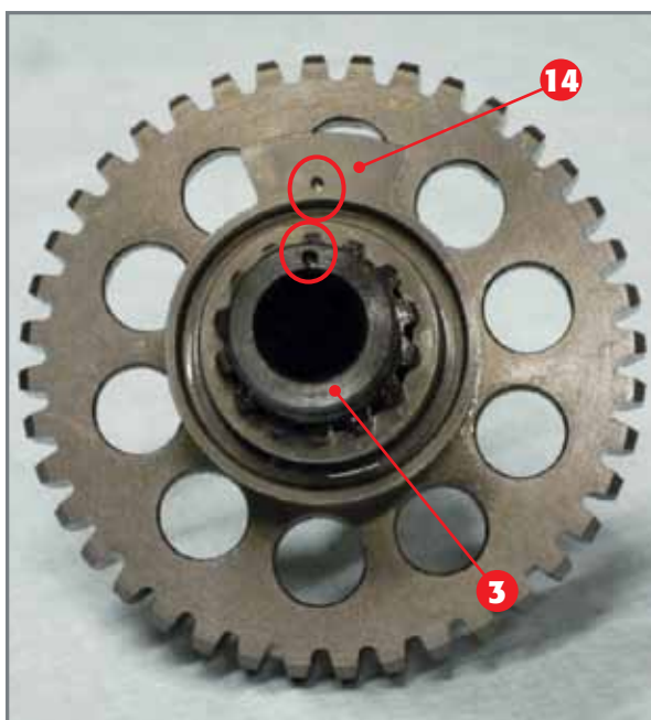
Positionierung der Muffe auf der Welle.
