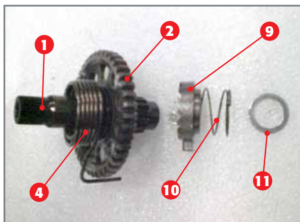
Der komplette Kickstarterwelle über Pedal
