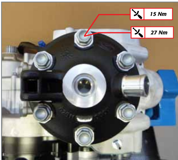
Anzug Zylinderkopf.
