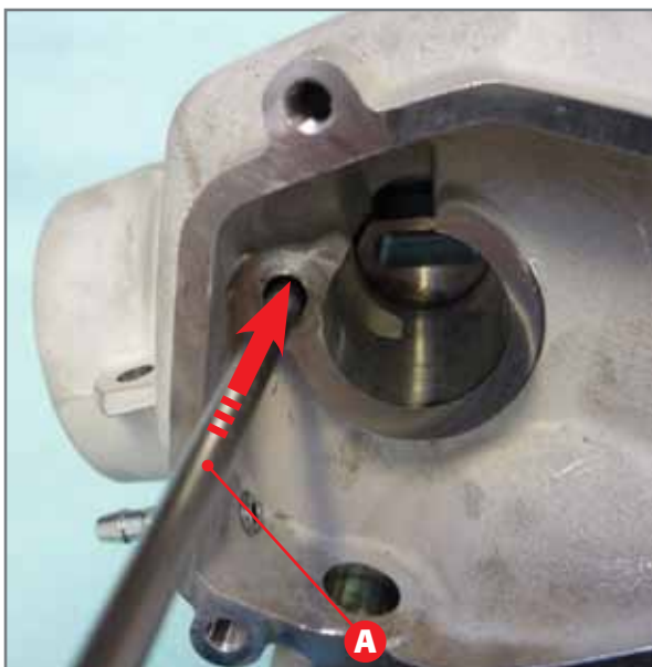
Herausziehen des Stiftes.
