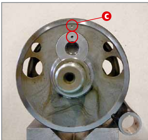
Markierungen C an Kurbelwangen und Hubzapfen.
