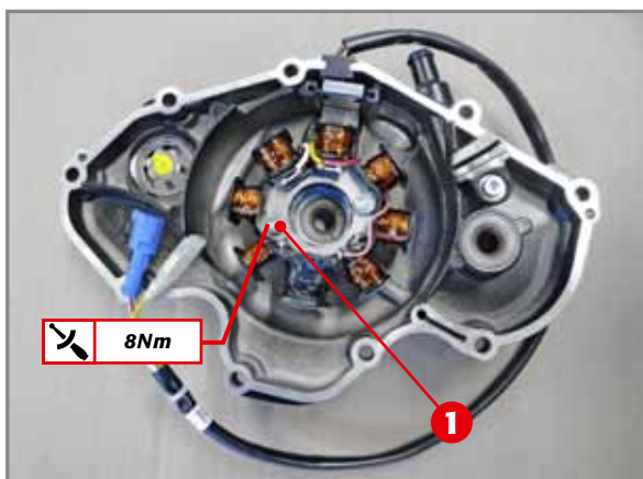
Anbringen des Stators am Zündungsdeckel.
