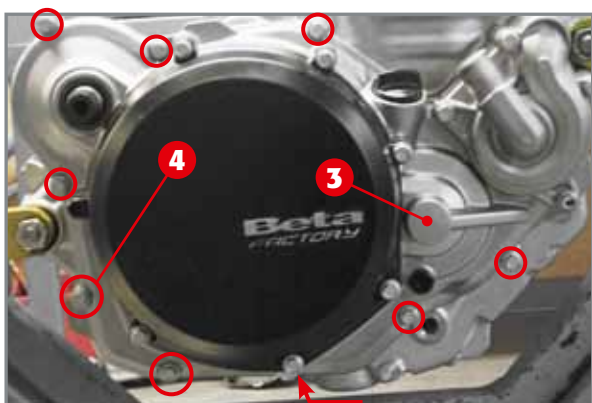
Der innere Kupplungsdeckel 3 und die entsprechenden Schrauben 4.
