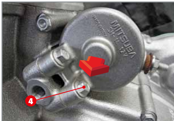
Die beiden Schrauben C, die den Anlasser am Gehäuse befestigen.
